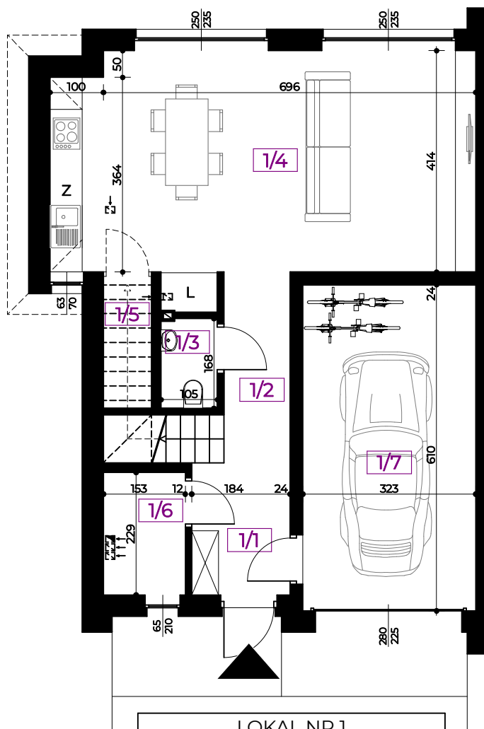
RZUT PARTERU 1:100
