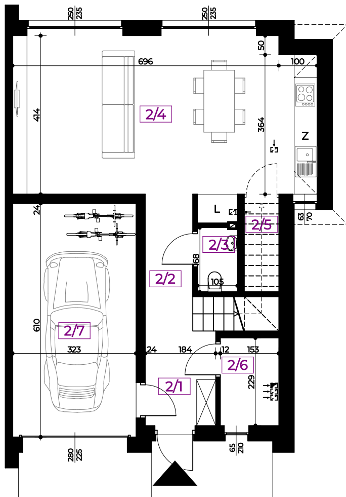
RZUT PARTERU 1:100
