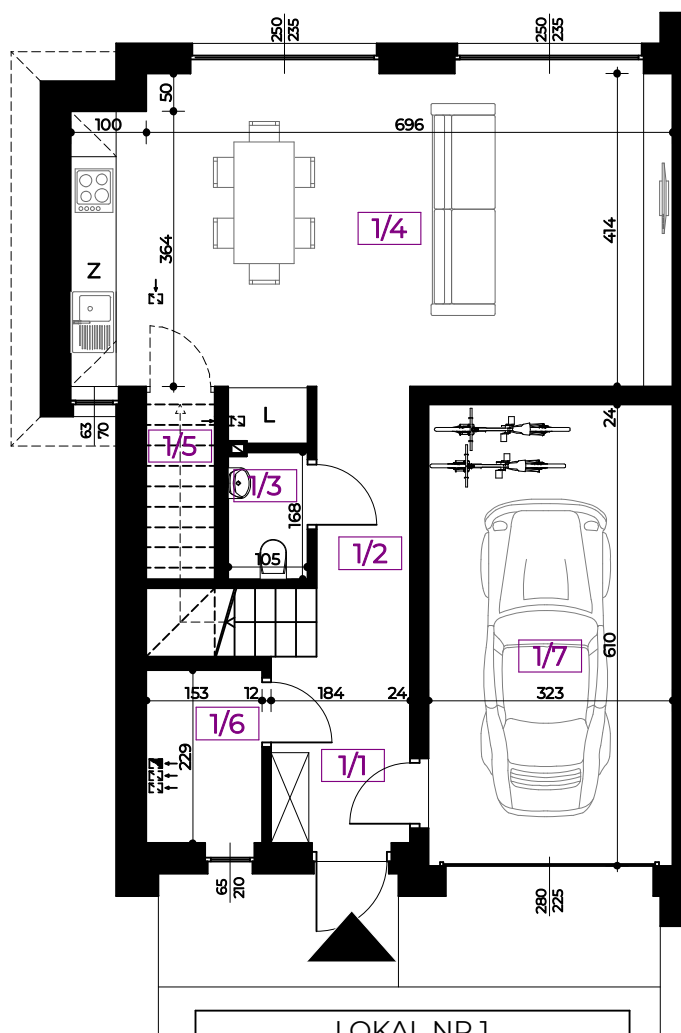
RZUT PARTERU 1:100
